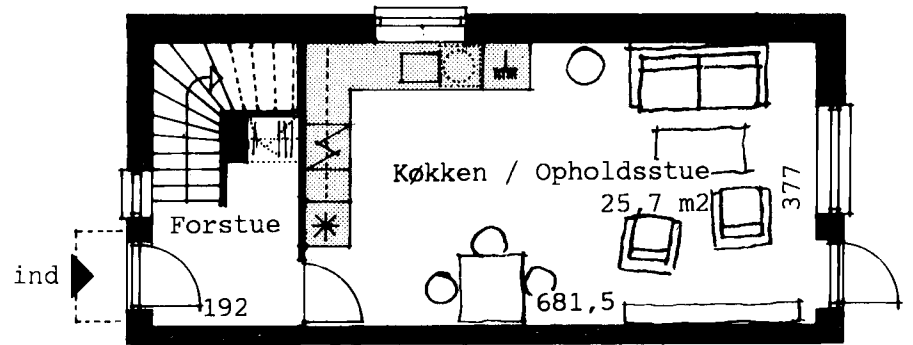
Stueplan
