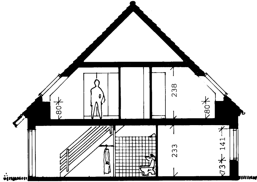
Tværsnit
