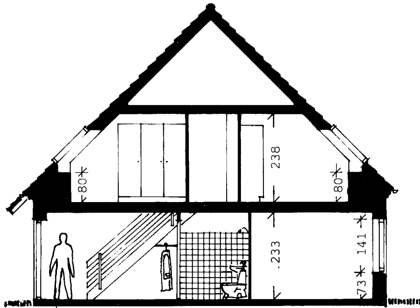
Tværsnit
